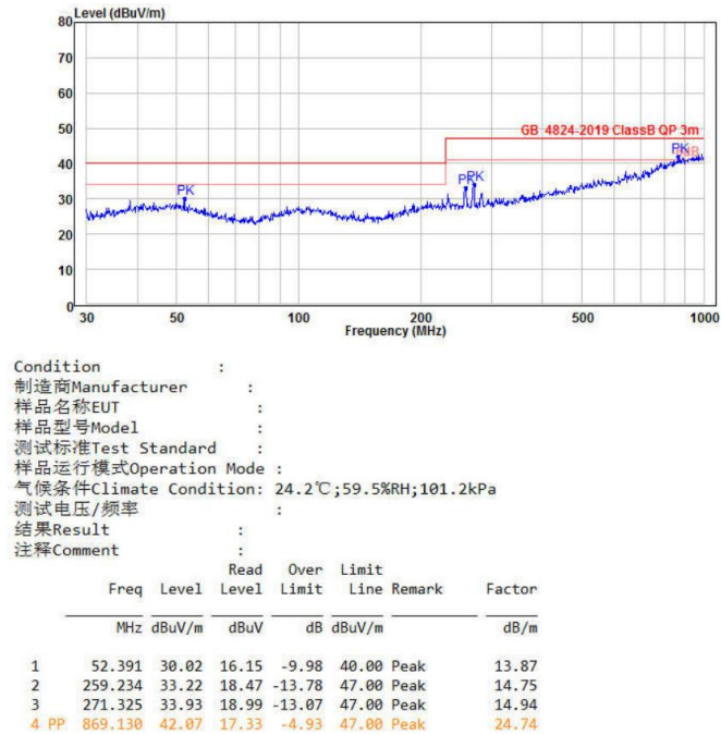
图 5-5 RE 测试水平方向
