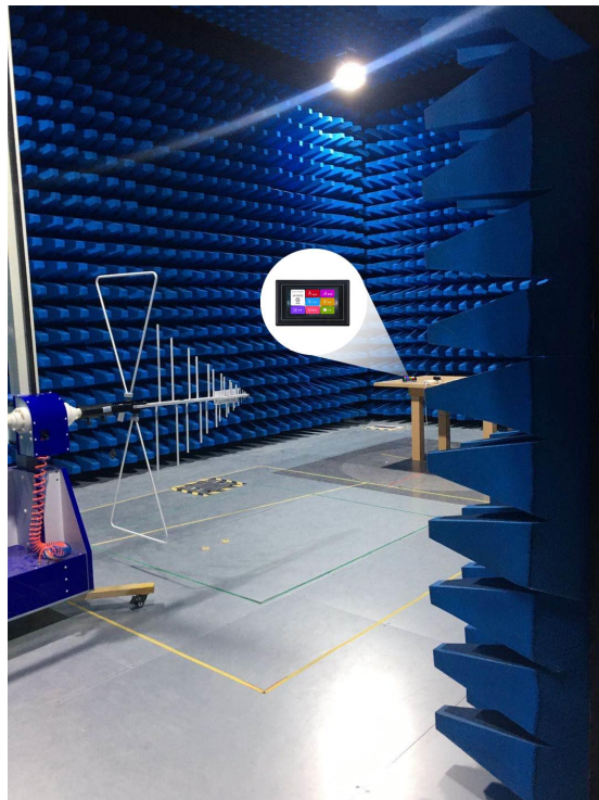
图 5-4 RE 测试图
